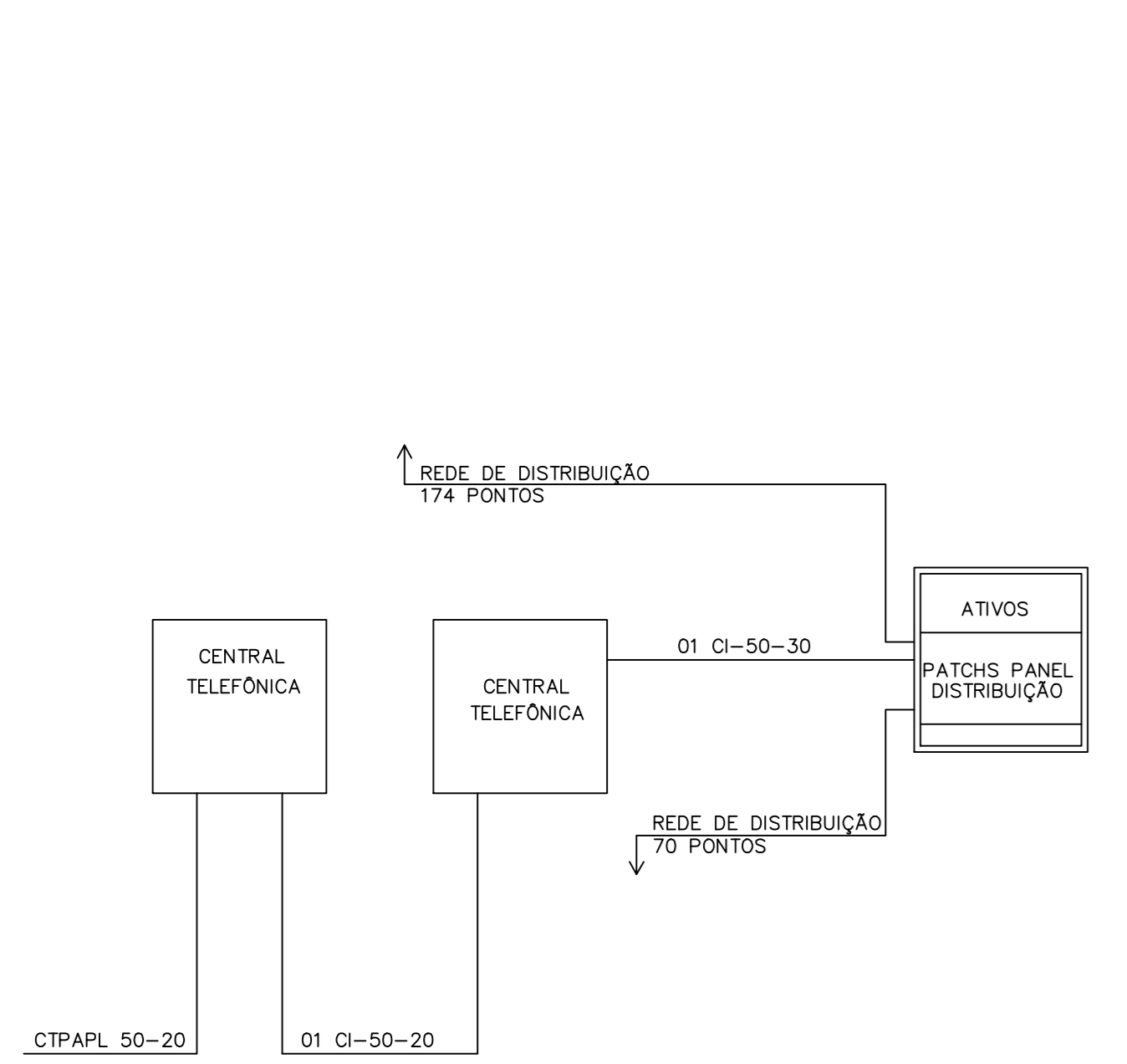
DIAGRAMA DA REDE ESTRUTURADA SEM ESCALA
