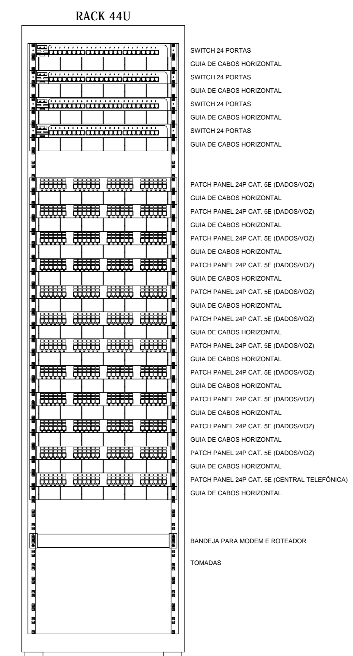
DETALHE DO RACK SEM ESCALA
