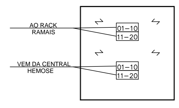
DETALHE DISTRIBUIDOR GERAL SEM ESCALA
