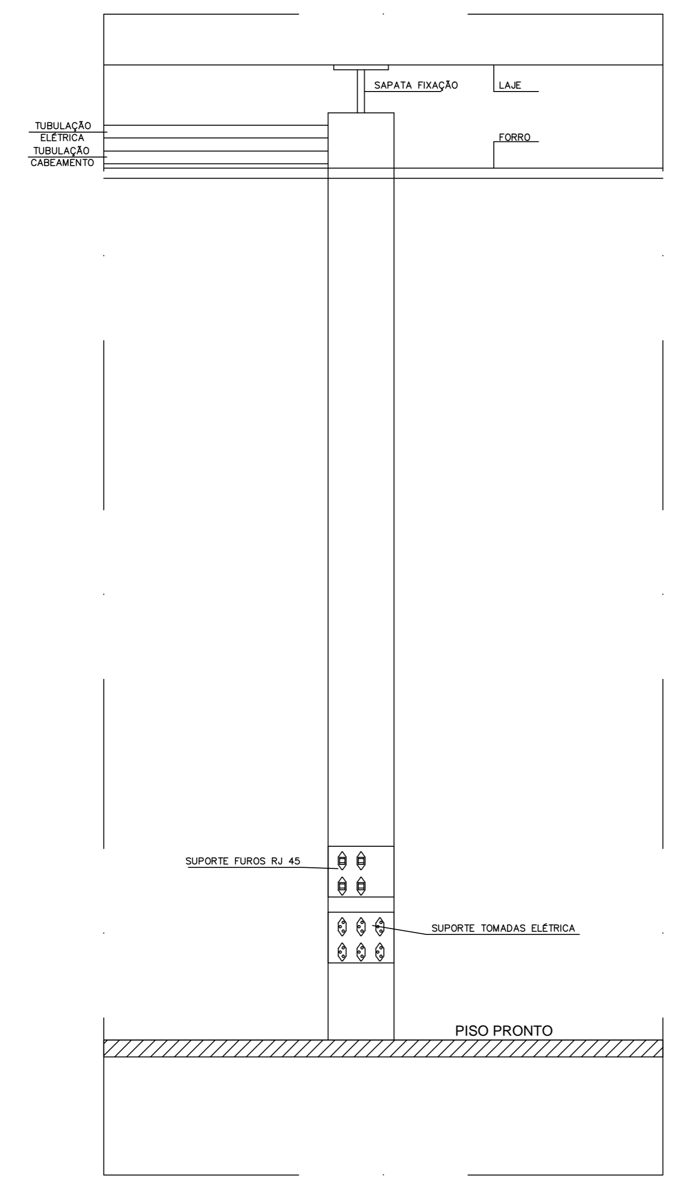
DETALHE DOS PONTOS NA ESQUADRIA/PILARES SEM ESCALA
