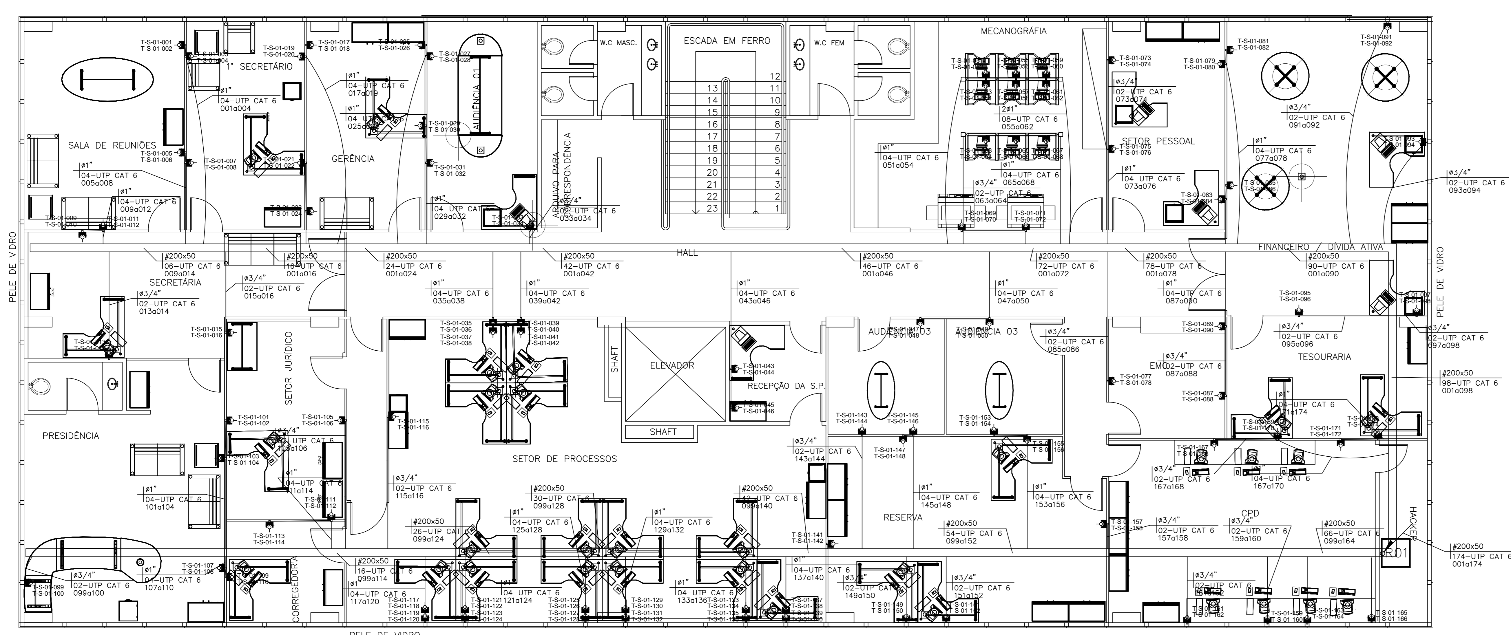
PLANTA BAIXA SUPERIOR REDE LOCAL ESCALA 1/75
