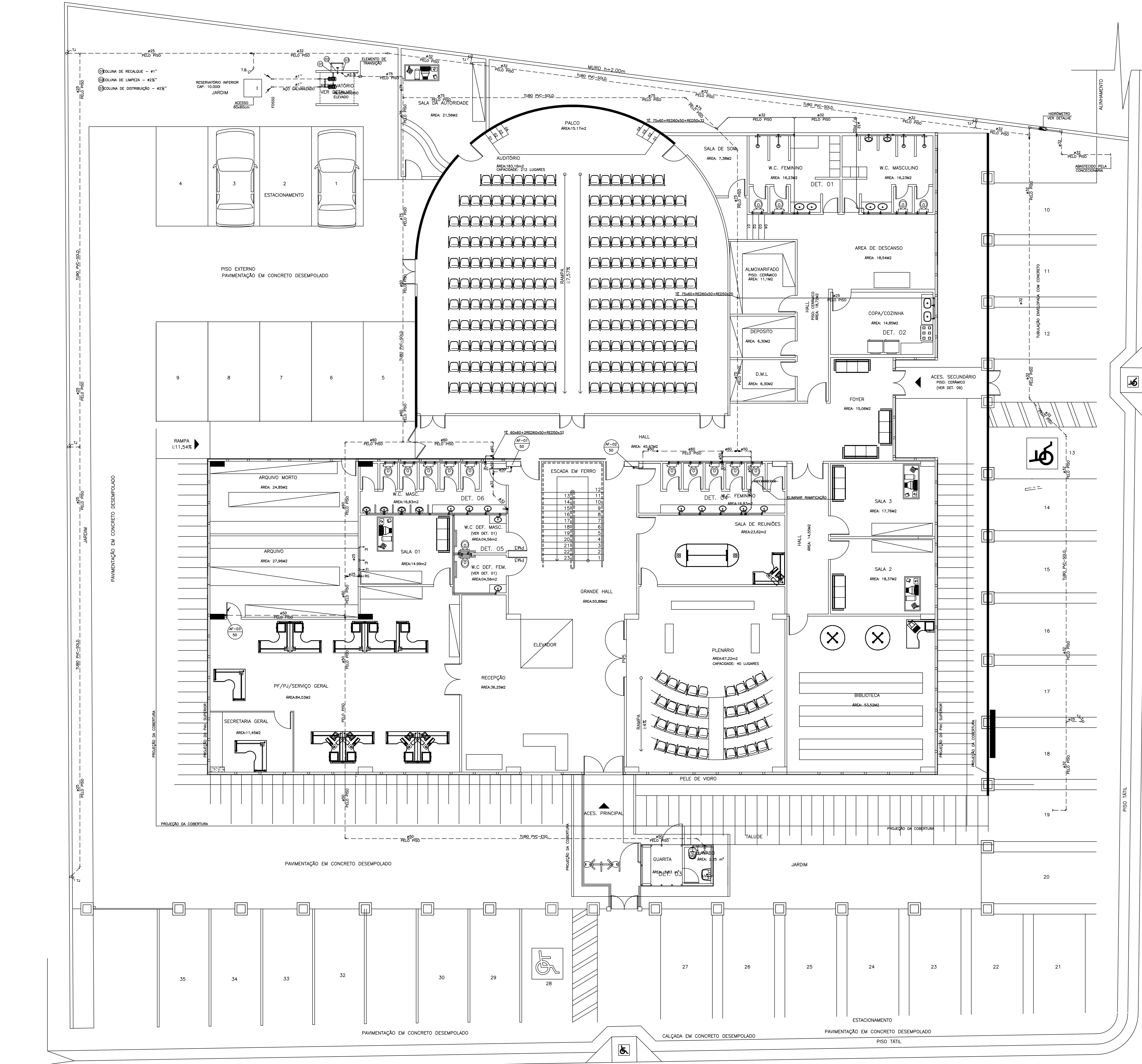
PLANTA BAIXA TÉRREO ESCALA 1/75
